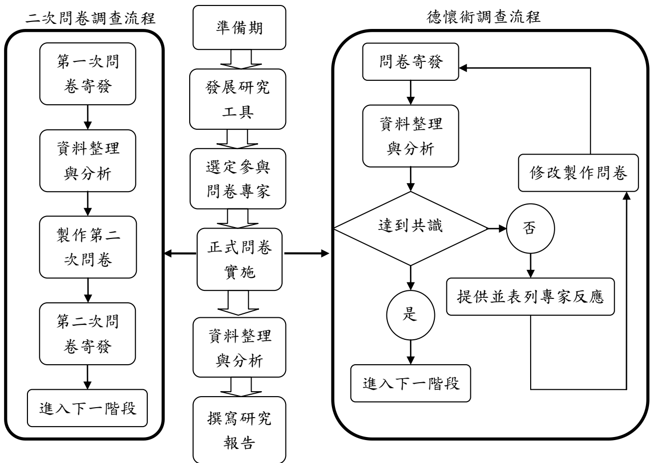
圖 1 研究流程圖
