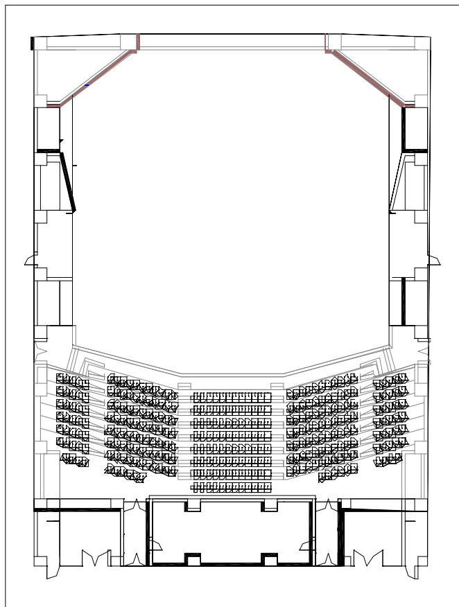
大學館演藝廳三、四樓座椅平面圖 ( 330 席 )
