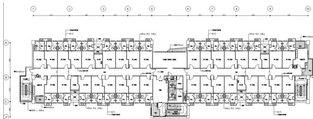
圖 5.7 標準層平面圖
