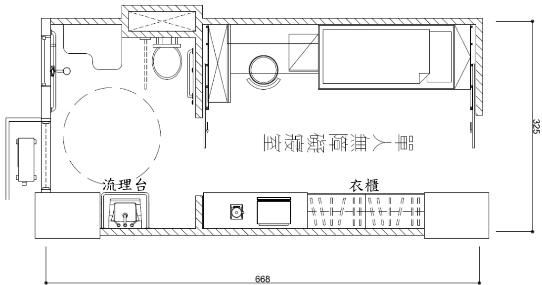
圖 5.10 單人無障礙宿舍空間單元平面圖
