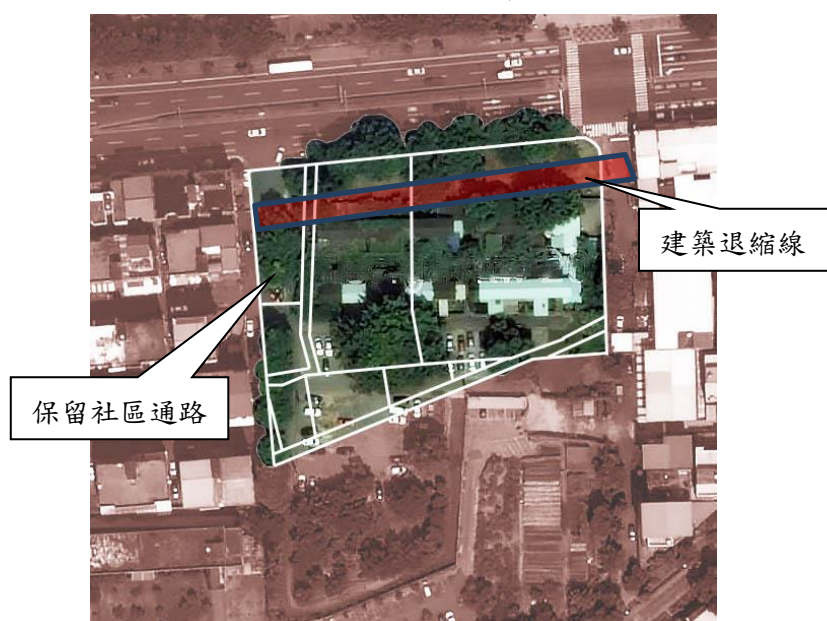
圖 5.2 現況地籍套繪及建物退縮位置圖
