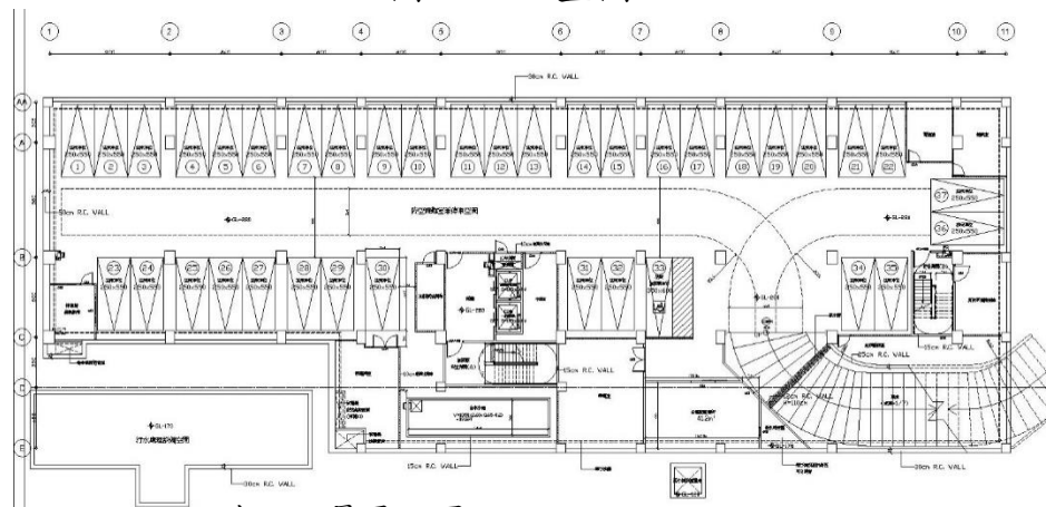
圖 5.5 配置圖
