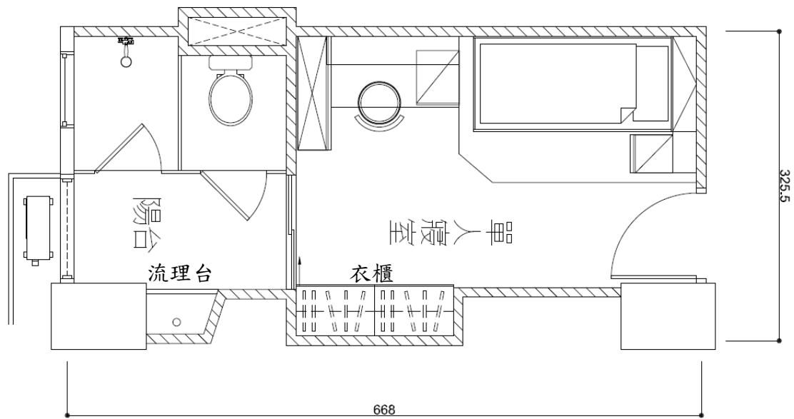
圖 5.9 單人宿舍空間單元平面圖
