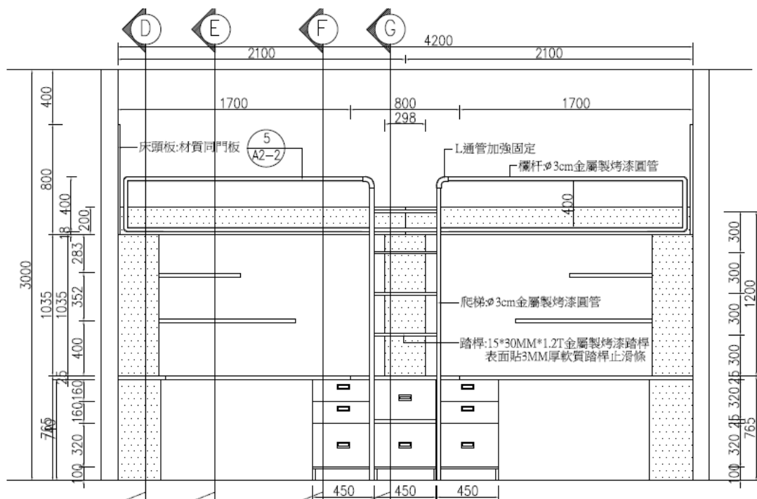
圖 5.8 學生宿舍空間單元平立面圖
