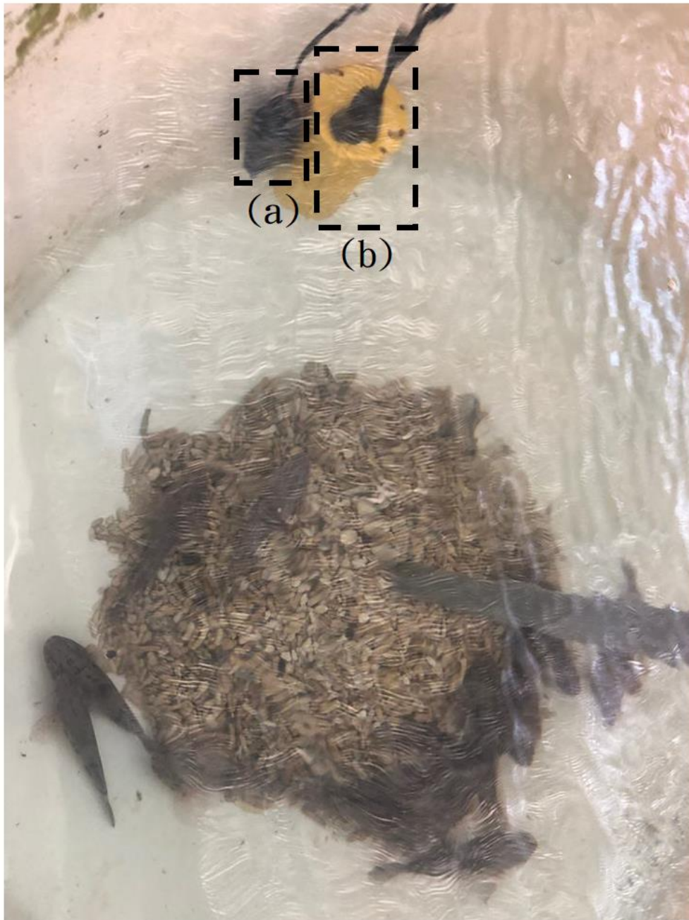
圖一、(a)PH 感測器 (b)DO 與溫度感測器
